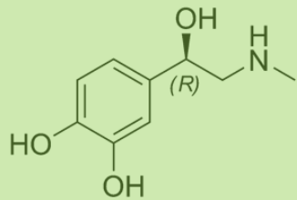
adrénaline
