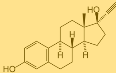
éthinyloestradiol
