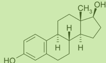
estradiol
