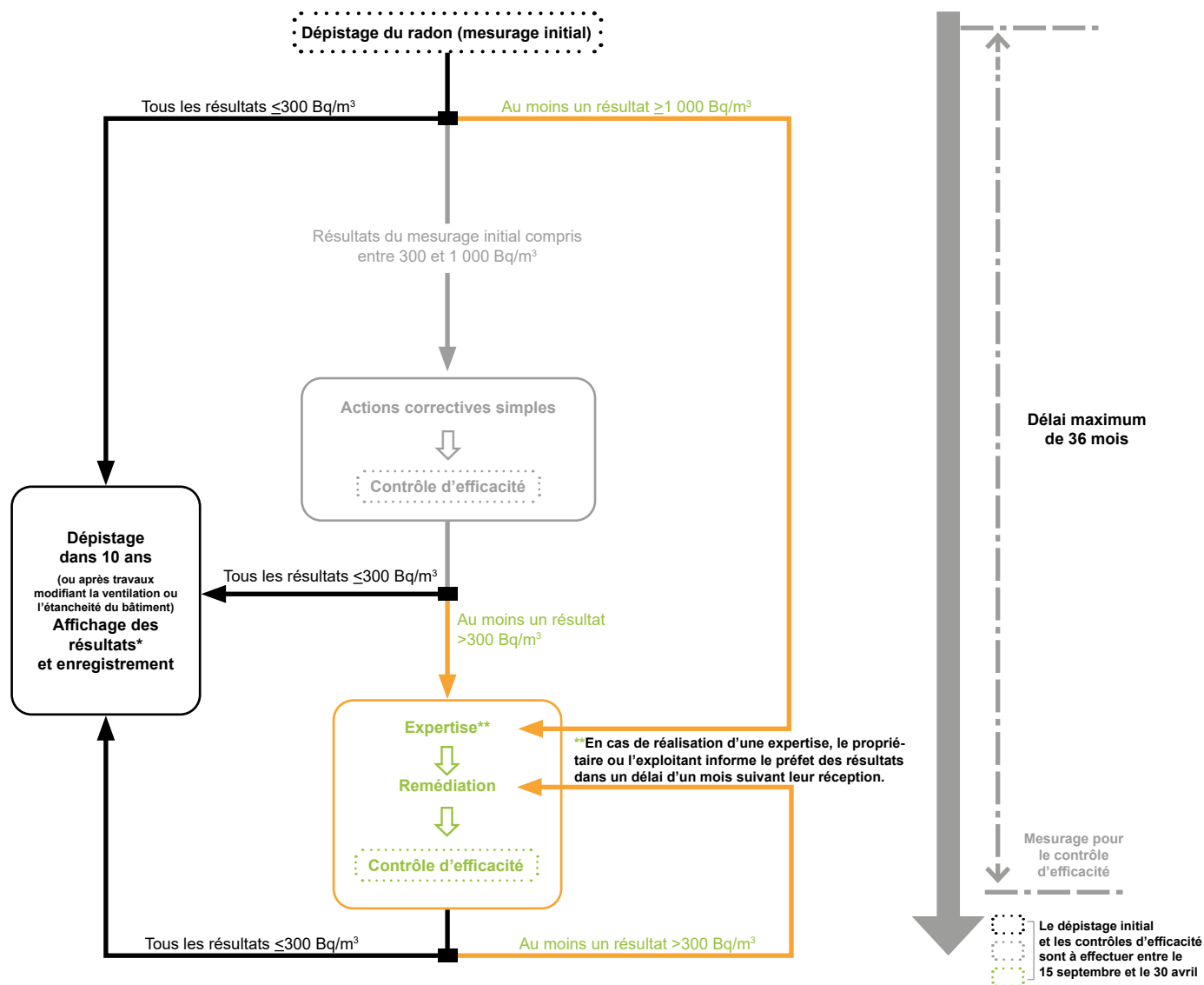
Figure 2 : modalités de gestion du radon dans les ERP en zone 3 et dans les ERP en zones 1 et 2 disposant de résultats de mesurages antérieurs au 01/07/2018 supérieur à 300 Bq/m 3 (source : Autorité de sûreté nucléaire).
