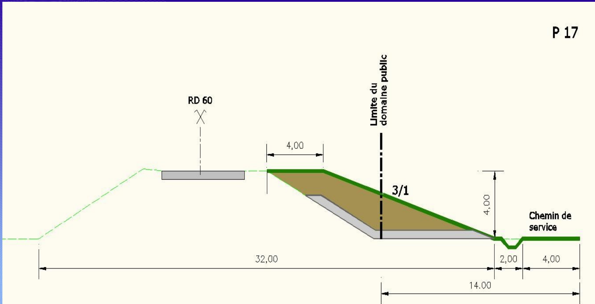
Principe du renforcement côté val
