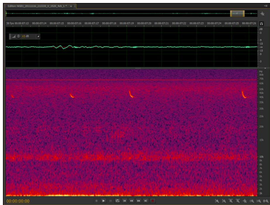
Figure 13 : Exemple de fichier son collecté sur le système d'enregistrement TrackBat.
