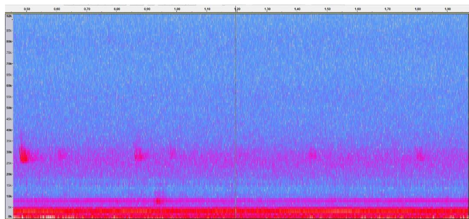
Figure 27 : Sonogramme de cris émis par une Sérotine commune
