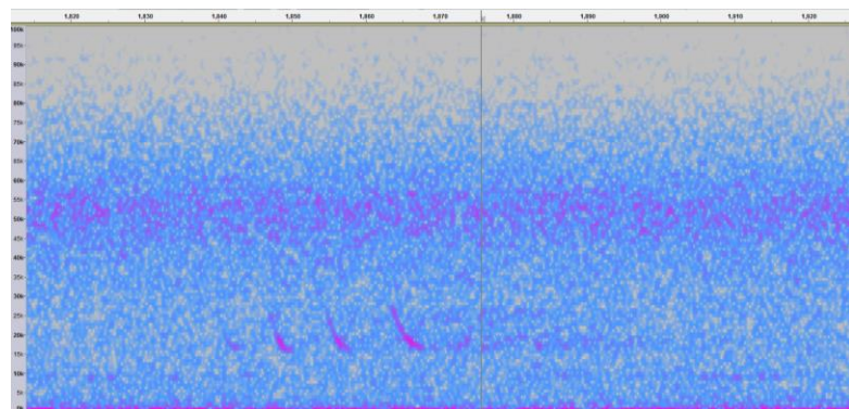
Figure 23 : Sonogramme de cris émis par une Noctule commune
