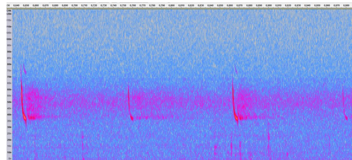
Figure 20 : Sonogramme des cris de Pipistrelle de Nathusius/Kuhl
