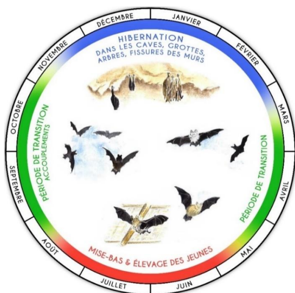
Figure 28 : Cycle biologique des chiroptères, LPO Touraine
