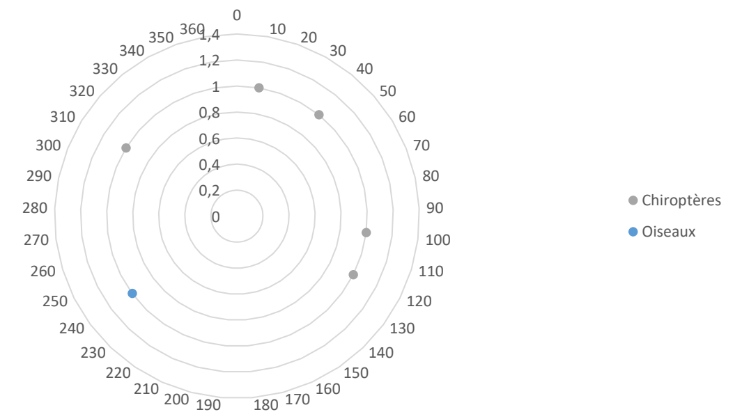
Graphique 5 : Répartition des cadavres en fonction de l'orientation par rapport au mât, sur le parc éolien de Longchamp en 2020
