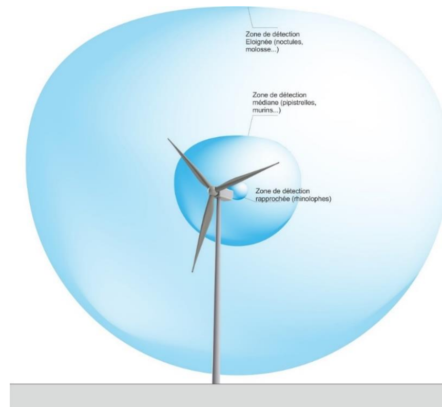
Figure 16 : Distance de détection des espèces de chauves-souris en fonction de leur fréquence d'émission
