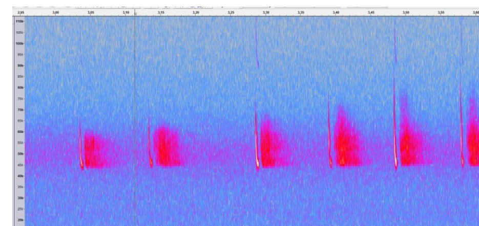
Figure 18 : Sonogramme de cris émis par une Pipistrelle commune
