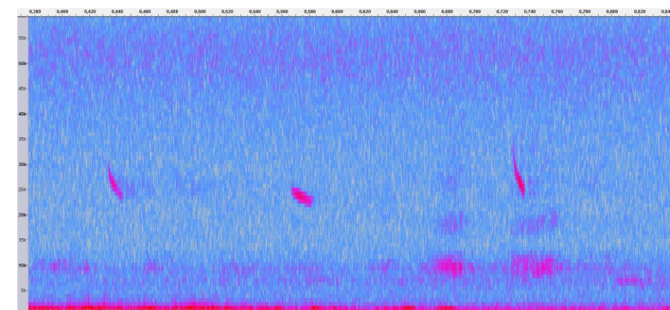
Figure 25 : Sonogramme de cris émis par une Noctule de Leisler
