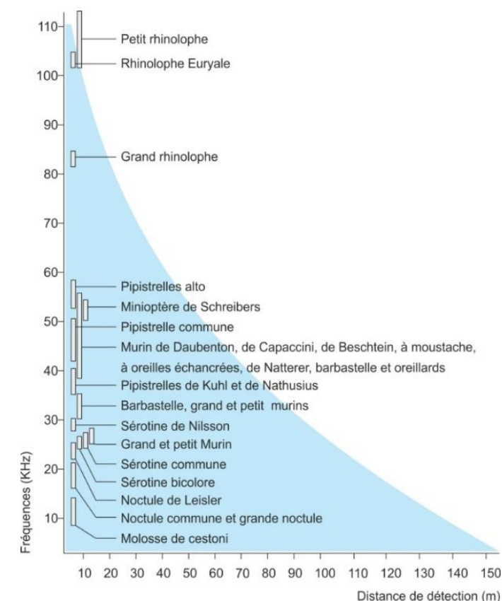
Figure 15 : Représentation des volumes de détection en fonction des groupes d'espèces
