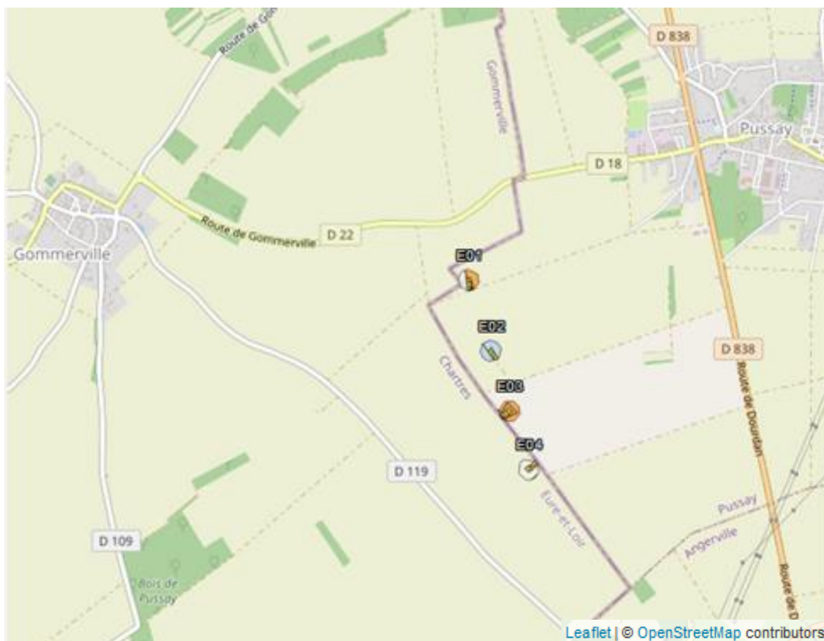
Figure 3 : Situation et disposition des éoliennes du parc éolien des Vingt Sétiers 2 (CEVIN II)
