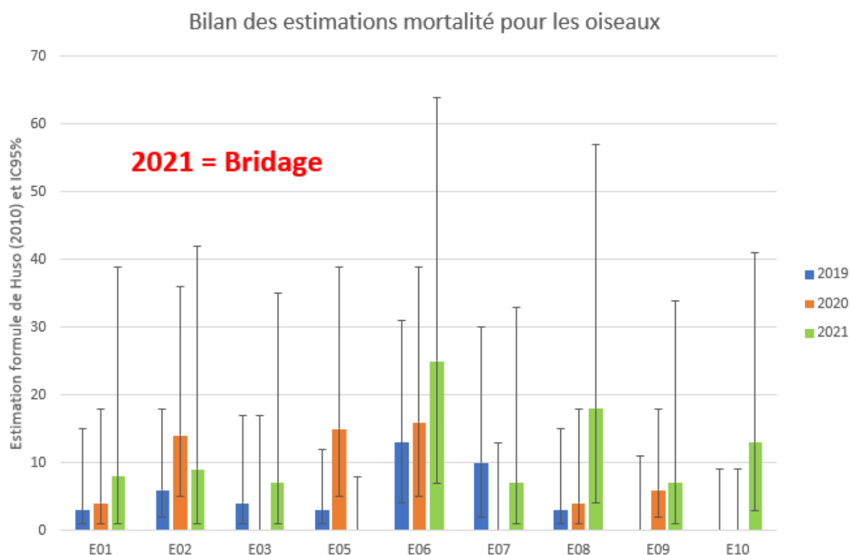
Figure 72 : Bilan de la mortalité probable (et intervalle de confiance à 95%) pour les suivis 2019, 2020 et 2021 pour le parc éolien de Chassepain pour l'avifaune
