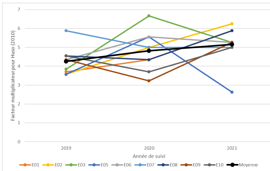
Figure 59 : Evolution du facteur multiplicateur de la formule de Huso (2010) pour les 9 éoliennes lors des suivis 2019, 2020 et 2021
