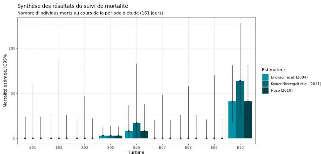
Figure 63 : Estimation de la mortalité la plus probable (et incertitude à 95%) pour les chiroptères pour le parc éolien de Chassepain au cours du suivi de 2021 sur 161 jours
