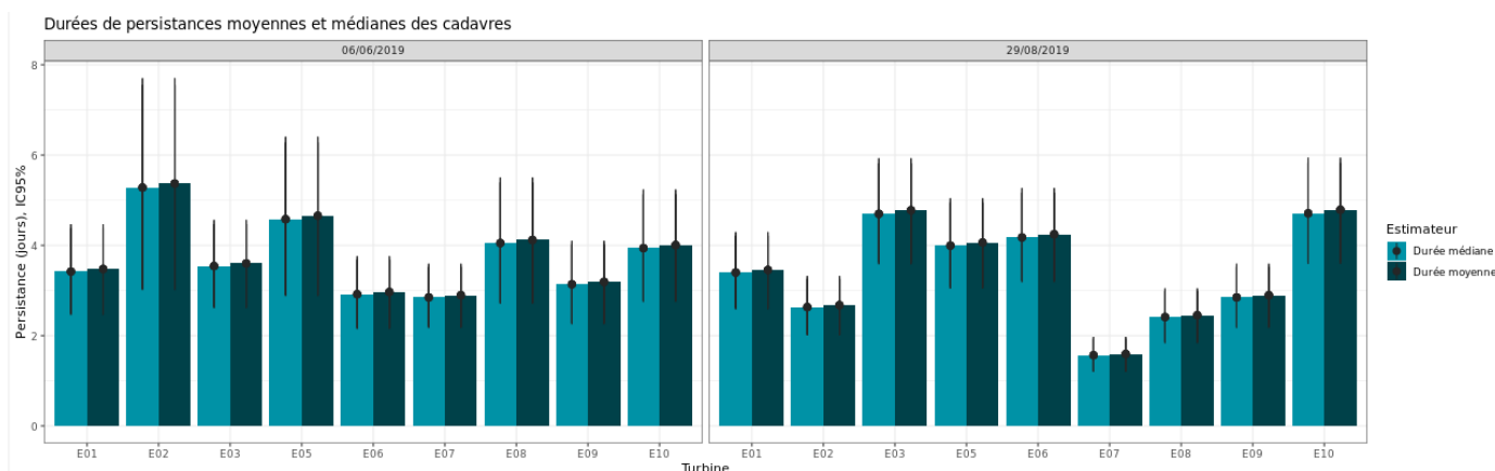
Figure 54 : Durées de persistance moyennes des cadavres et incertitudes (intervalles de confiance à 95%)
