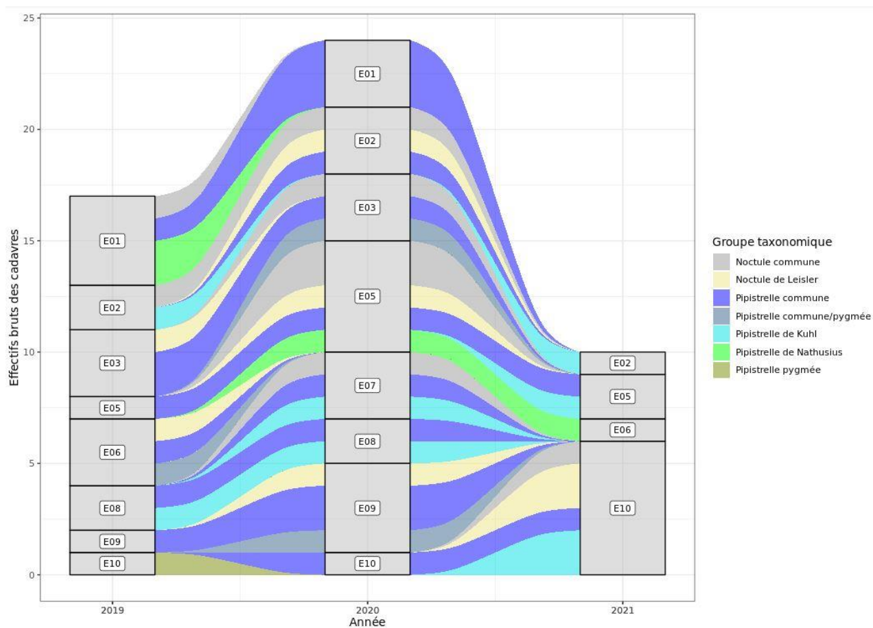
Figure 53 : Evolution de la mortalité des chiroptères selon les années sur le parc éolien de Chassepain
