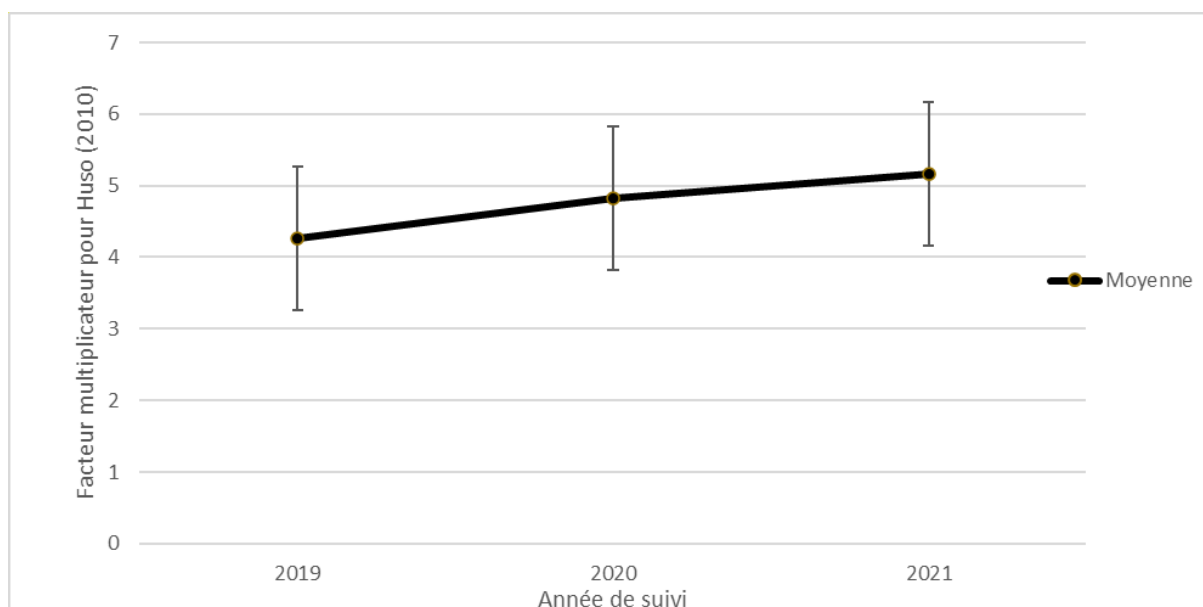
Figure 60 : Evolution de la moyenne du facteur multiplicateur de la formule de Huso (2010) pour les 9 éoliennes lors des suivis 2019, 2020 et 2021
