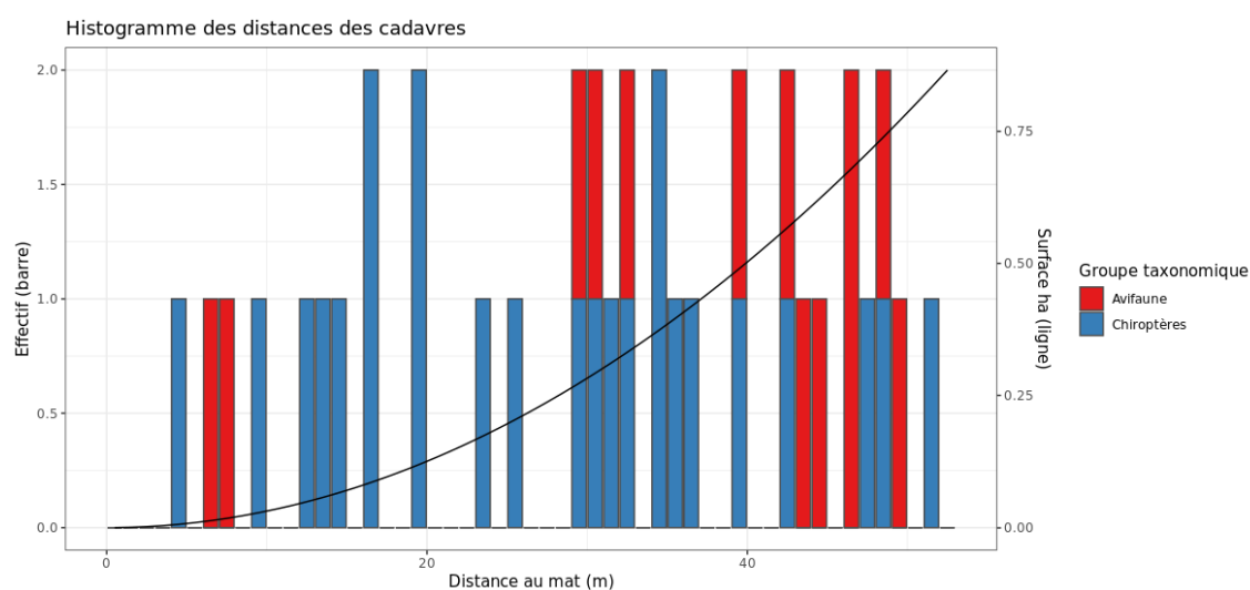
Figure 48 : Répartition spatiale (distance à l'éolienne) des cadavres retrouvés au sein du parc de Chassepain en 2020. La courbe représente l'évolution de la surface de l'aire d'étude prospectée en fonction de la distance au pied de l'éolienne.
