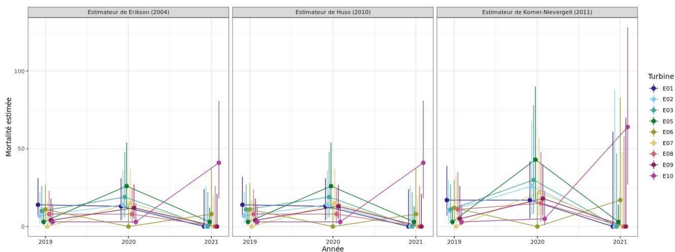
Figure 65 : Bilan de la mortalité probable (et intervalle de confiance à 95%) pour les suivis 2019, 2020 et 2021 pour le parc éolien de Chassepain pour les chiroptères
