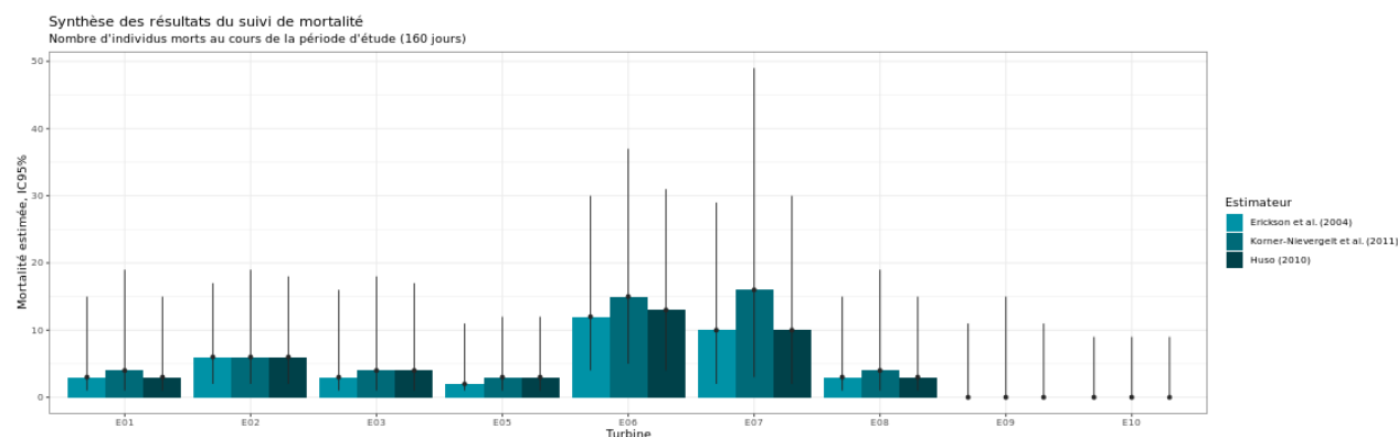
Figure 67 : Estimation de la mortalité la plus probable (et incertitude à 95%) pour les oiseaux pour le parc éolien de Chassepain au cours du suivi de mai à octobre 2019
