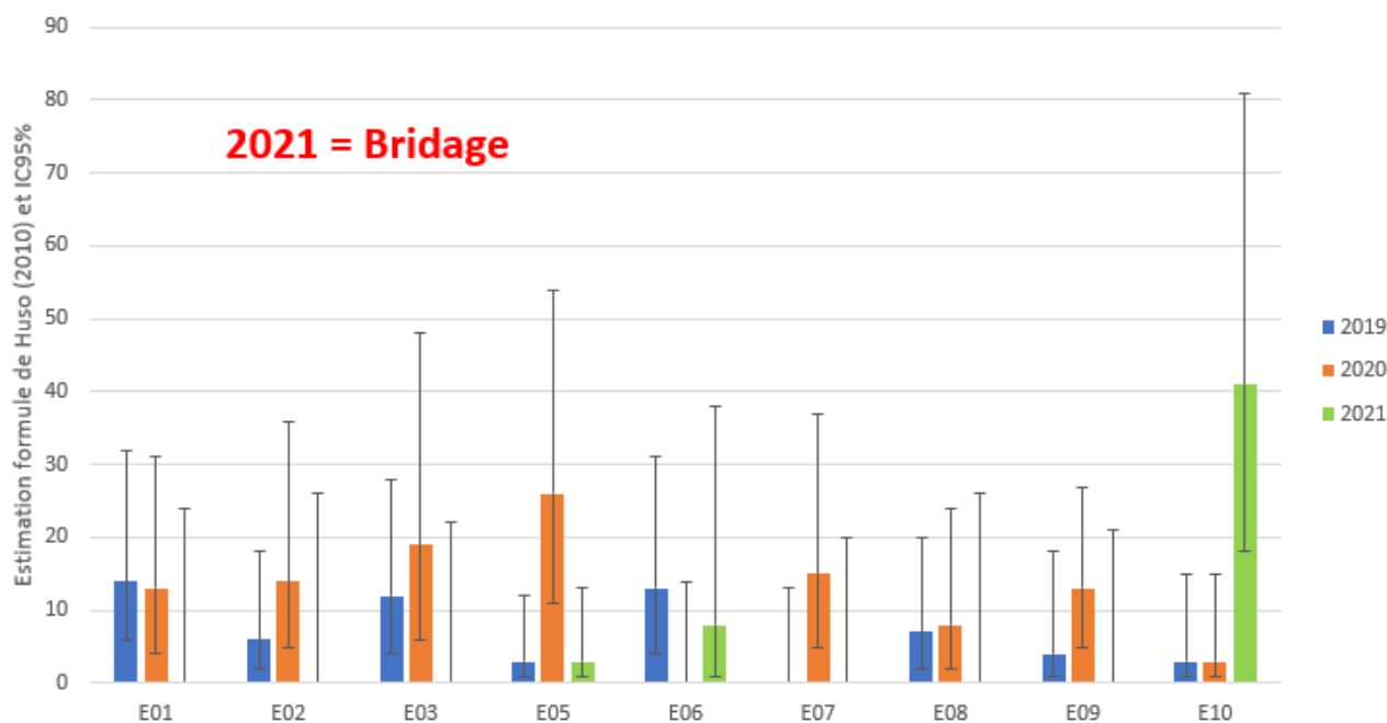
Figure 66 : Bilan de la mortalité probable (et intervalle de confiance à 95%) pour les suivis 2019, 2020 et 2021 pour le parc éolien de Chassepain pour les chiroptères
