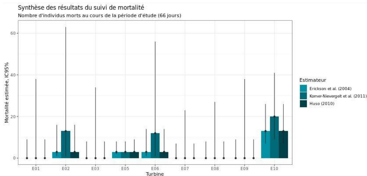
Figure 64 : Estimation de la mortalité la plus probable (et incertitude à 95%) pour les chiroptères pour le parc éolien de Chassepain au cours du suivi de 2021 sur 66 jours
