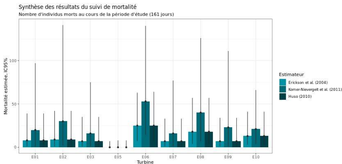
Figure 69 : Estimation de la mortalité la plus probable (et incertitude à 95%) pour les oiseaux pour le parc éolien de Chassepain au cours du suivi de 2021 sur 161 jours
