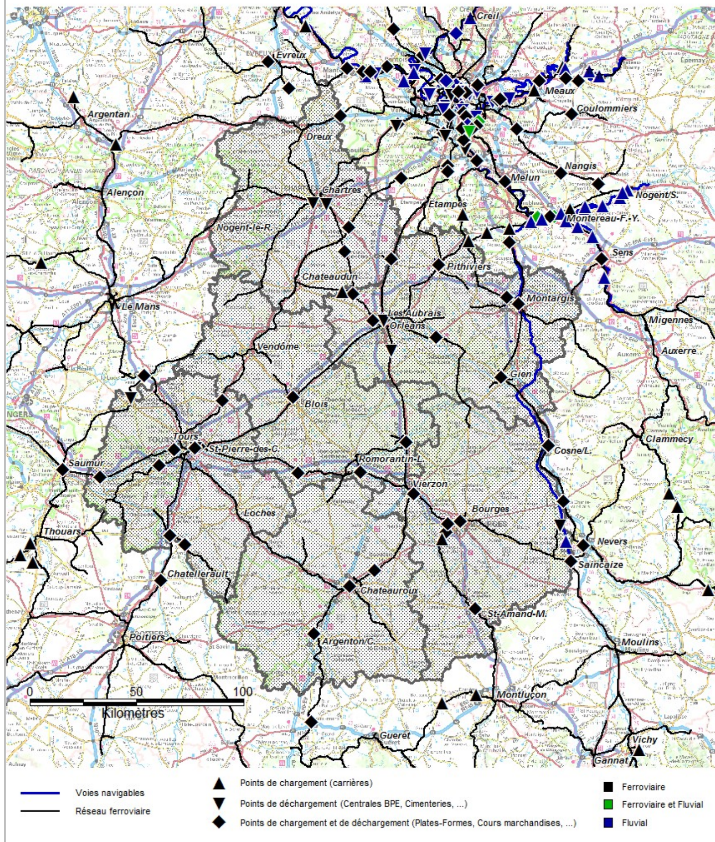
Infrastructures ferroviaires et fluviales mobilisables pour transporter les produits de carrières en 2015
