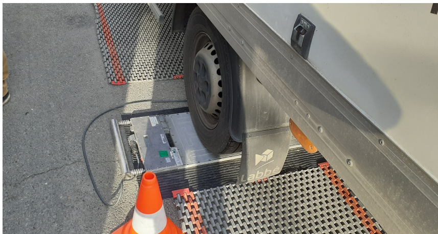
Pesée d'un véhicule de transport léger sur l'opération de contrôle de CHARTRES RD910 le 29/11/2023
